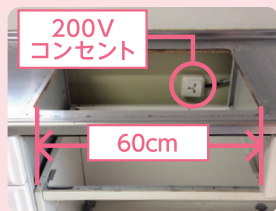
ガスコンロを枠から外して 単相200Vコンセントを設置
